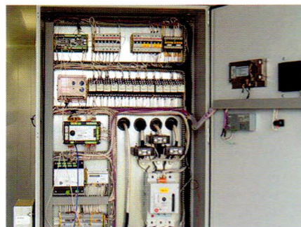
Щит управления газопоршневой (газовой) электростанцией. Третья степень автоматизации
