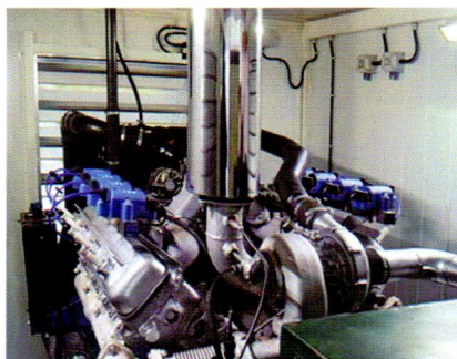
Газопоршневая (газовая) электростанция мощностью 200 кВт в блок-контейнерном исполнении
